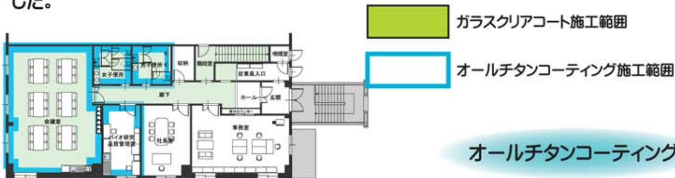
2階平面図
